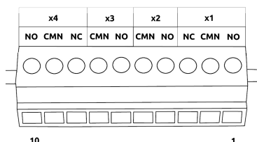
Figure 3.1. Szablon opisu pinów dla modułu MOD-MINI-4R
