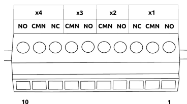
Figure 3.3. Szablon opisu pinów dla modułu MOD-MINI-4R
