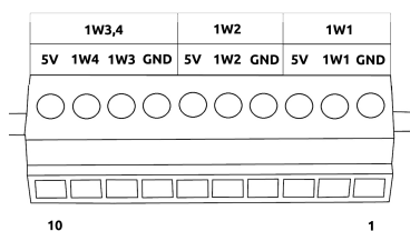
Figure 3.2. Szablon opisu pinów dla modułu MOD-MINI-4x1W
