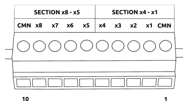
Figure 3.3. Szablon opisu pinów dla modułu MOD-MINI-8R
